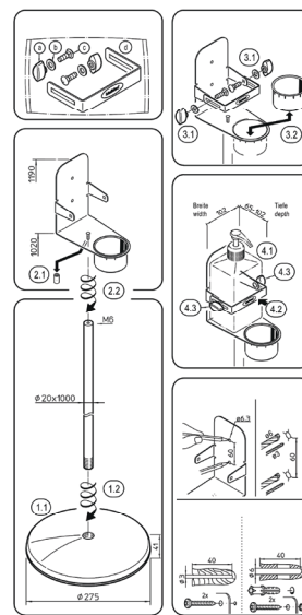
mit Klemmbügel
