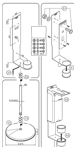
mit Lochbild
